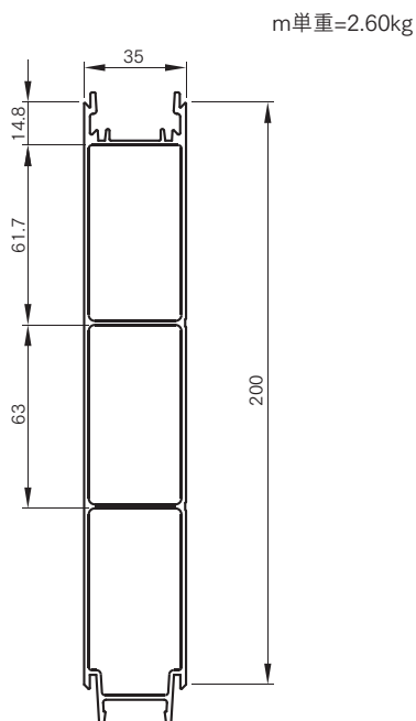
■(MTMA) 標準ミドル H=200
