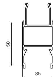
■(SMDZ) 50幅 ミドル H=50
