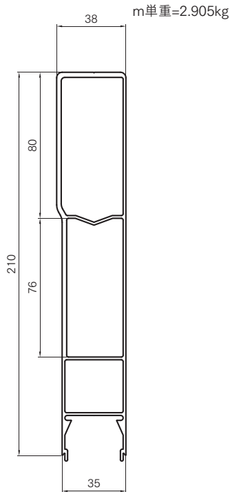
■(SUZ) 標準アッパー H=210
