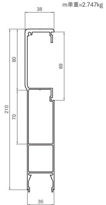
■(SUBZ) 2段用アッパー H=210
