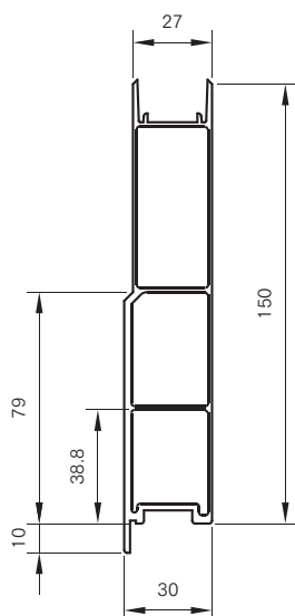
■(MLBA) 標準ボトム H=150
