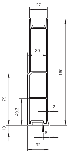
■(MLBK) FK用ボトム H=160
