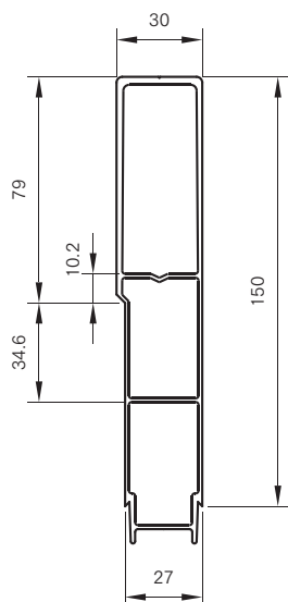
■(MLTA) 標準トップ H=150
