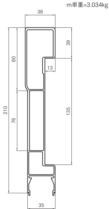
■(SUR) ラッシング用アッパー H=210
