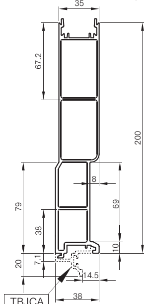
■(MTBJ) 外出し用ボトム H=200
