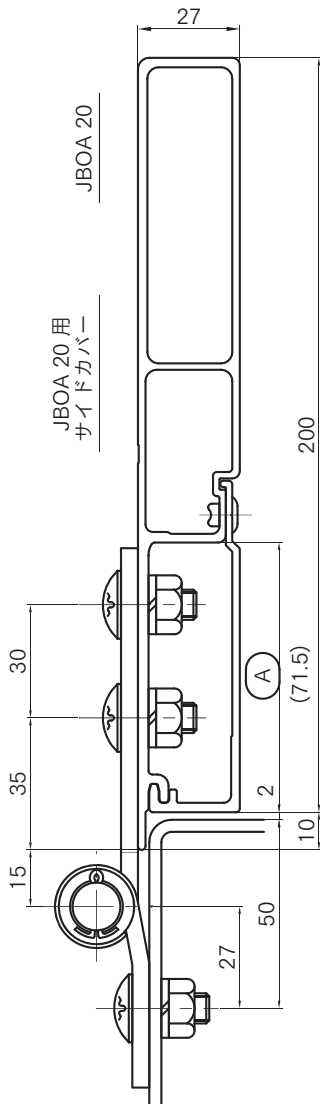
S型サイド蝶番を使用した組立例です
