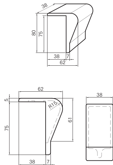
■(CB4) コーナーブロック
