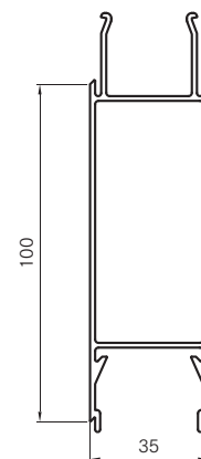
■(SMCZ) 100幅 ミドル H=100
