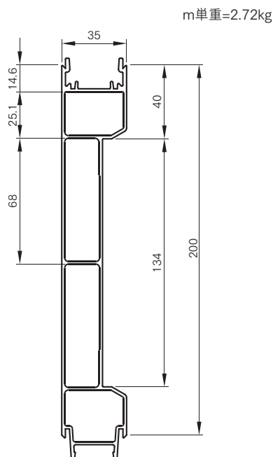
■(MTMR) ラッシング用ミドル H=200
