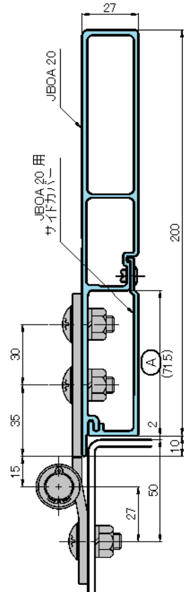
S型サイド蝶番を使用した組立例です
