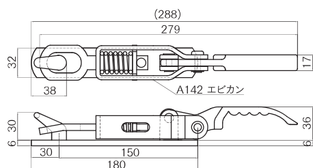
■鉄製 (6×32 座金付/A142エビカン付)
