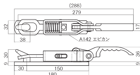
■鉄製 (9×32 座金付/A142エビカン付)
