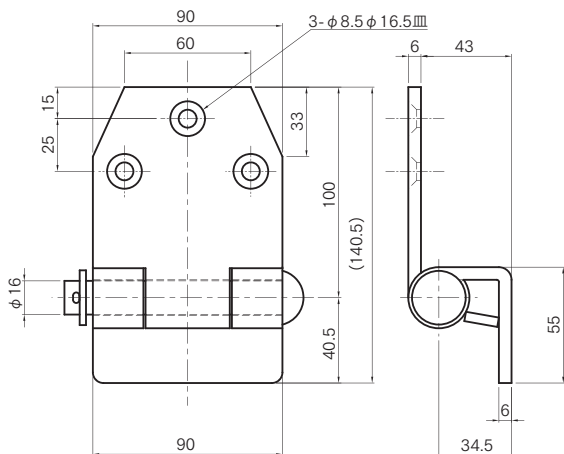
※図は右用を示す ※3価クロメートメッキ
