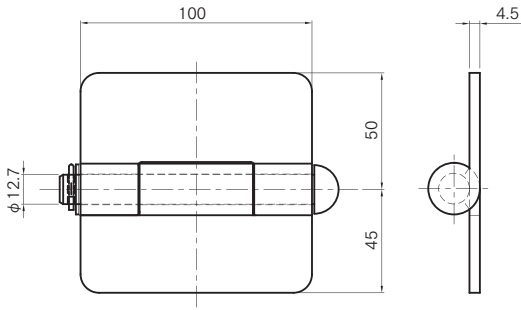
※図は右用を示す ※3価クロメートメッキ
