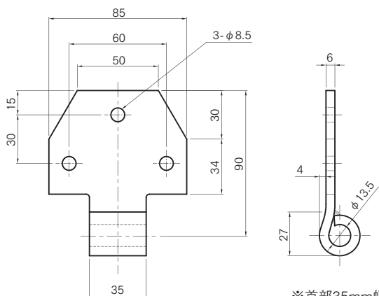
※首部35mm幅 ※3価クロメートメッキ
