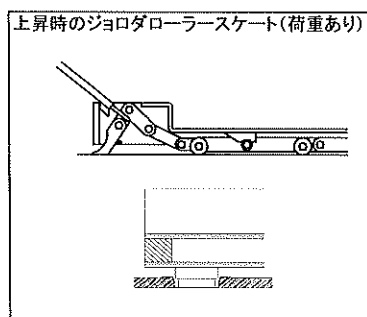
ジョロダローラースケートの仕様(能力) [ローリフト]
