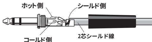
図 1 マイク及び予備入力プラグ
