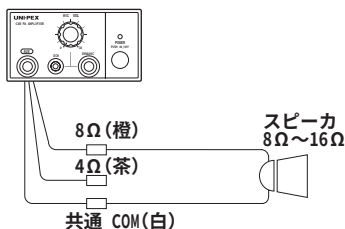
図 4 スピーカ接続例
