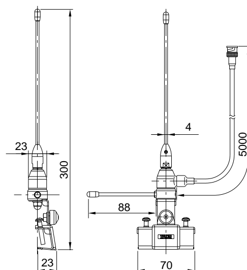
外観寸法図
