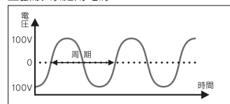
正弦波:家庭用電源
