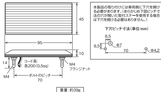
寸法 概寸(単位:mm)
